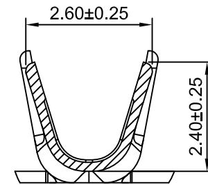
SEC:B-B
