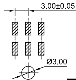
P.C.B LAYOUT (2x1P~2x3P)
