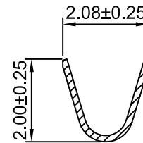
SEC:A-A
