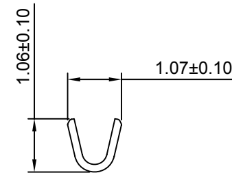
SEC:B-B
