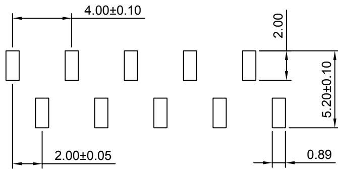
P.C.B LAYOUT
