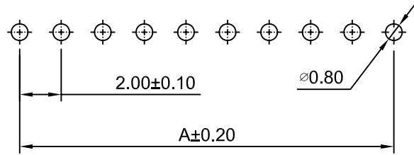
P.C.B LAYOUT
